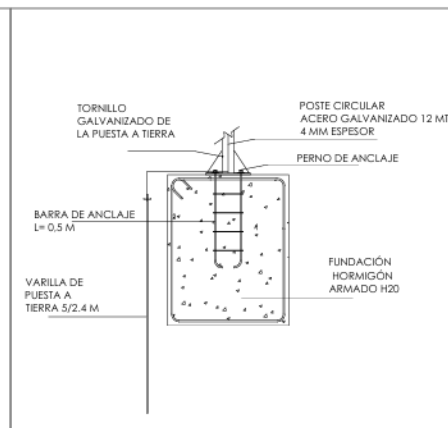
DETALLE 2. FUNDACIÓN 1/10
