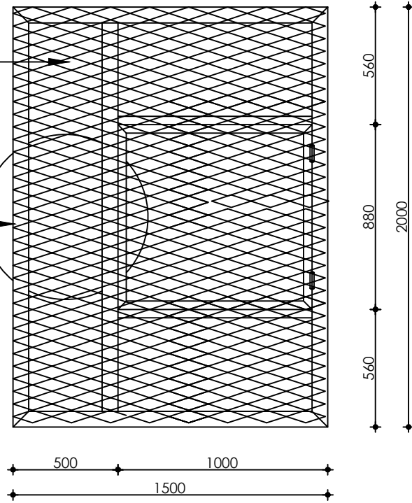
PLANTA ESC 1:25
