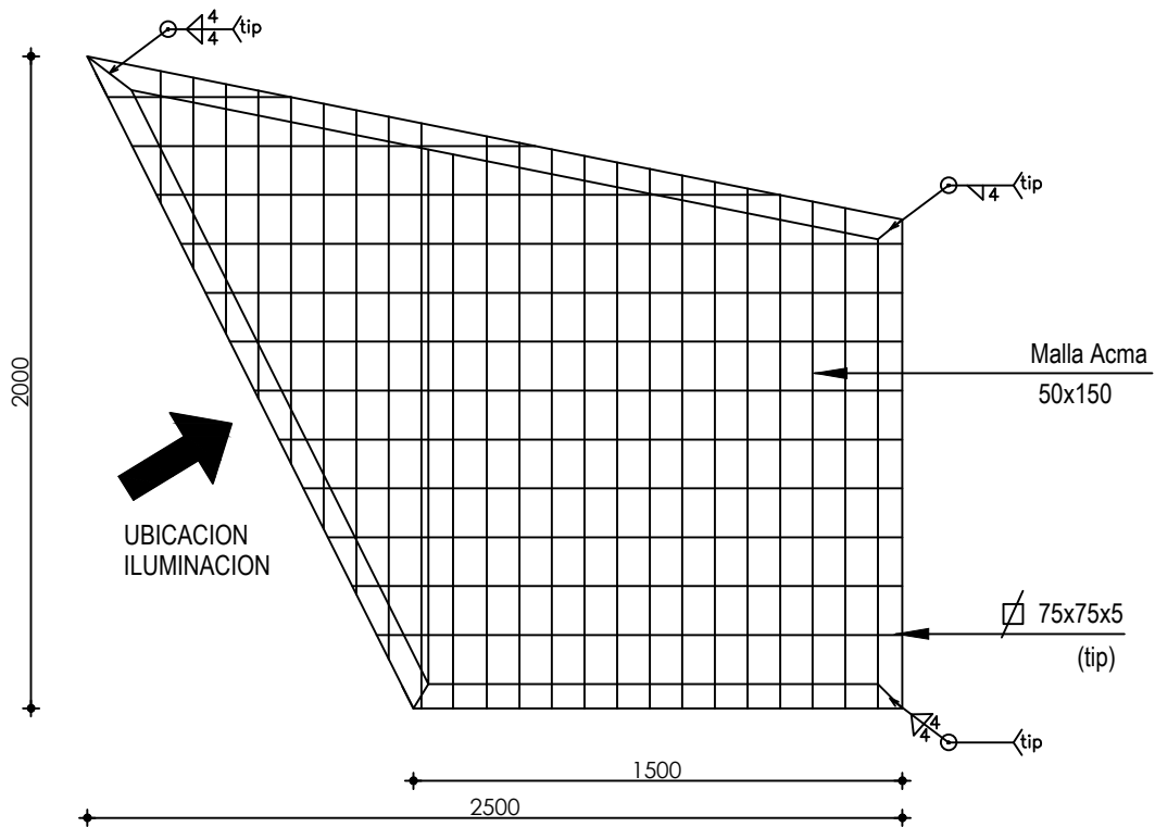
ELEVACION LATERAL ESC 1:25
